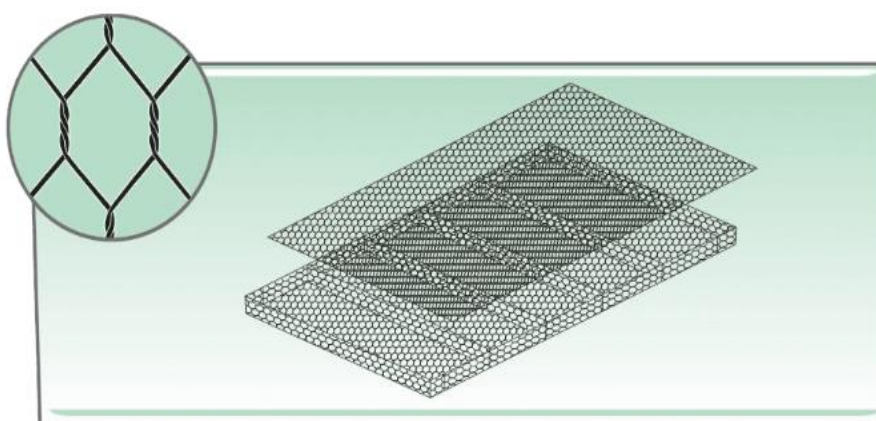
Figura 3 - Gabião colchão
